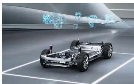
Модульная архитектура ARK
